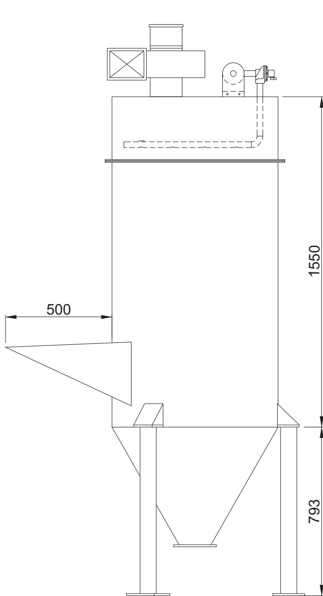
VISTA LATERAL
